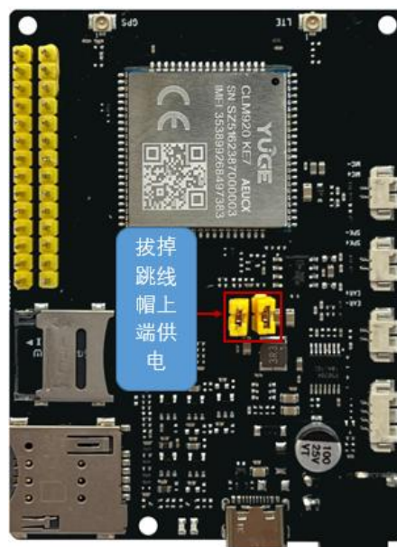
图 4-10 低功耗测试
