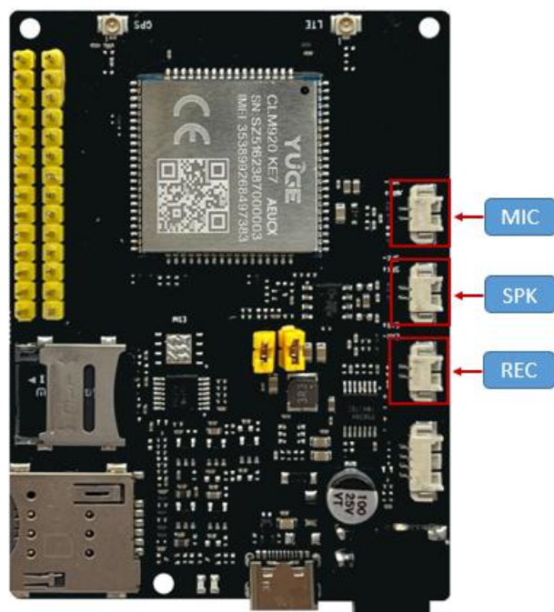
图 4-6 音频接口
