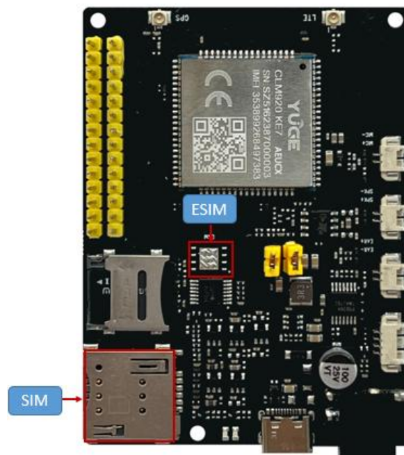
图 4-4 SIM 卡指示图
