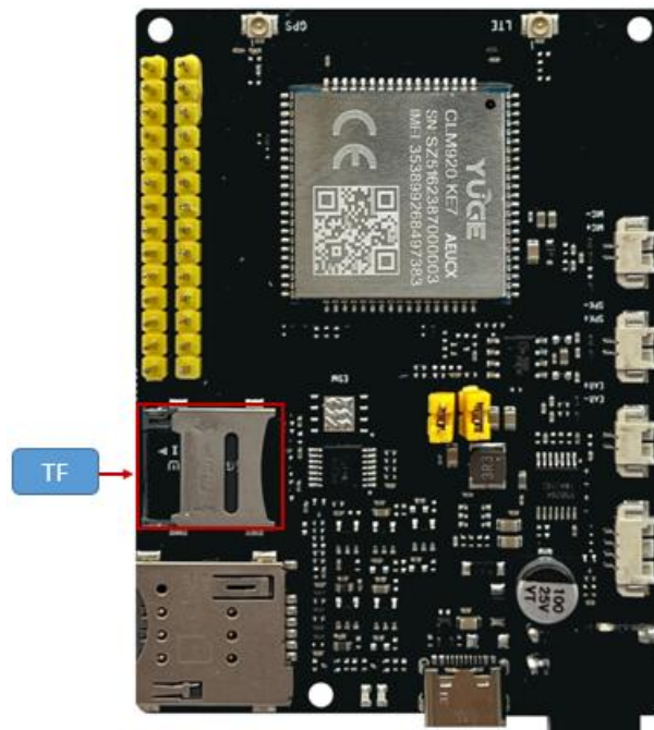
图 4-8 TF 卡接口
