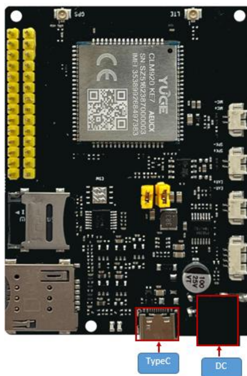
图 4-1 供电输入
