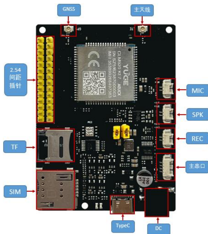
3-1 正面接口说明
