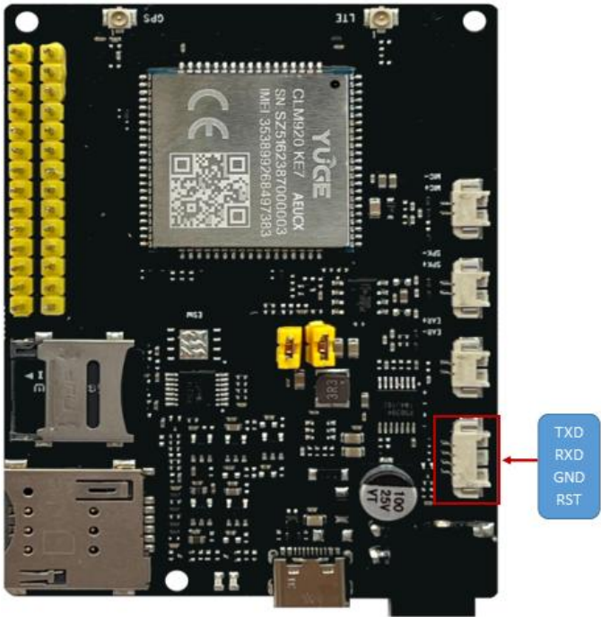
图 4-2 主串口指示图
