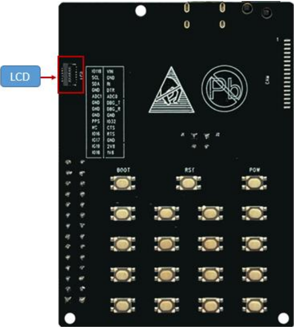
图 4-5 LCD 接口图
