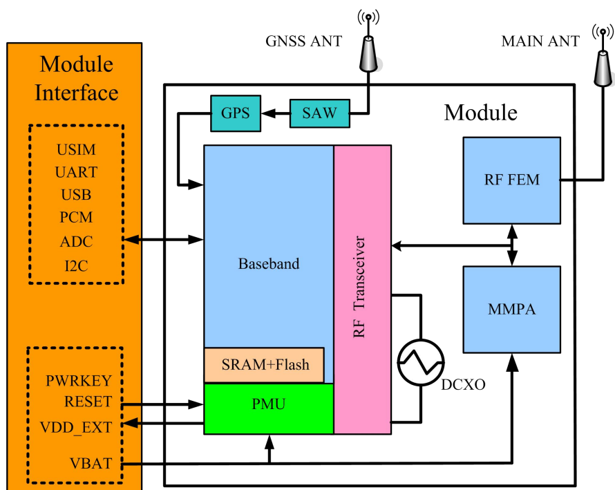
图 2-1 YM310 A09 模块功能框图
