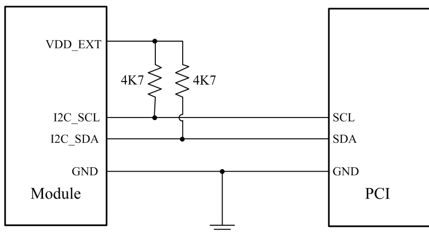
图 3-18 I2C 接口参考电路图
