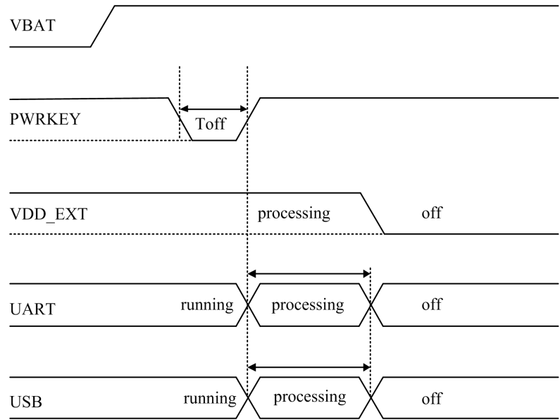
图 3-11 关机时序图
