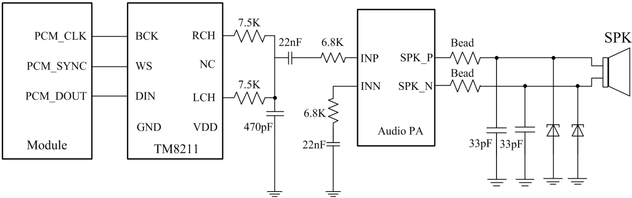
图 3-19 DAC 音频参考电路
