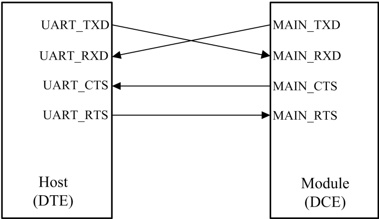
图 3-13 串口设计图
