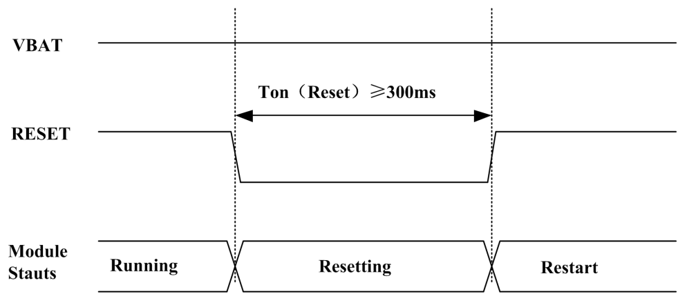
图 3-7 复位时序图
