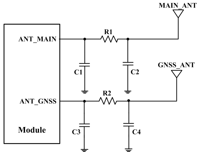
图 3-21 天线匹配电路
