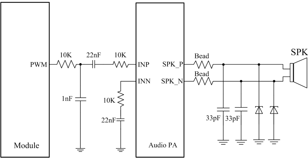
图 3-20 PWM 音频参考图
