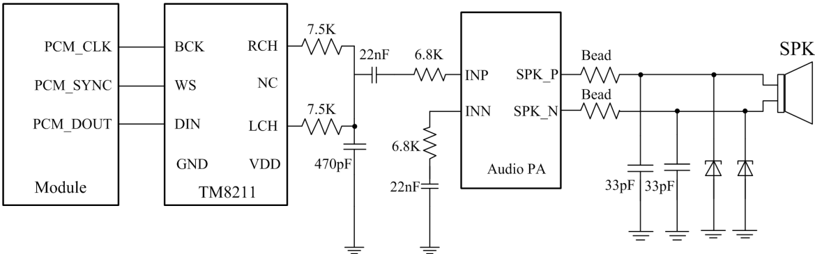
图 3-19 DAC 音频参考电路
