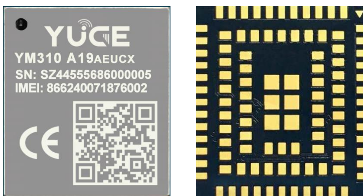
图 6-1 YM310 A19 外观图
