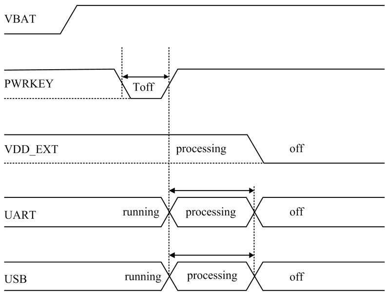
图 3-11 关机时序图
