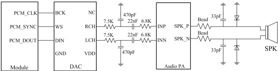
图 3-19 DAC 音频参考电路
