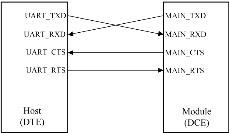
图 3-13 串口设计图
