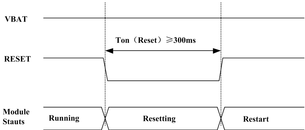
图 3-12 复位时序图
