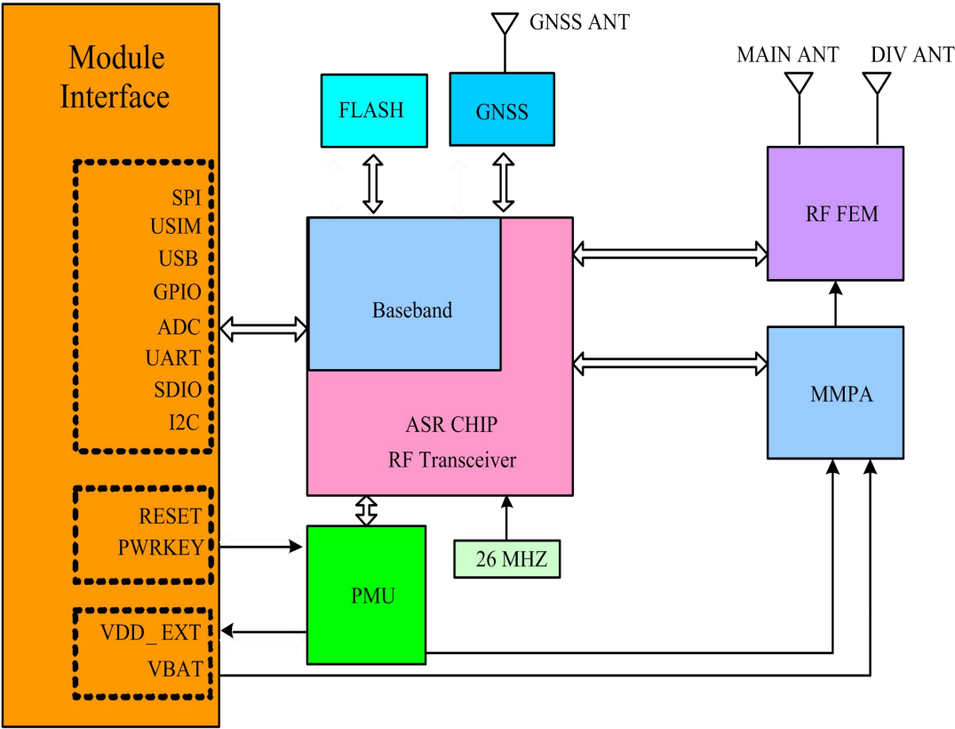
图2-1 CLM920 JC3F LCC模块功能框图
