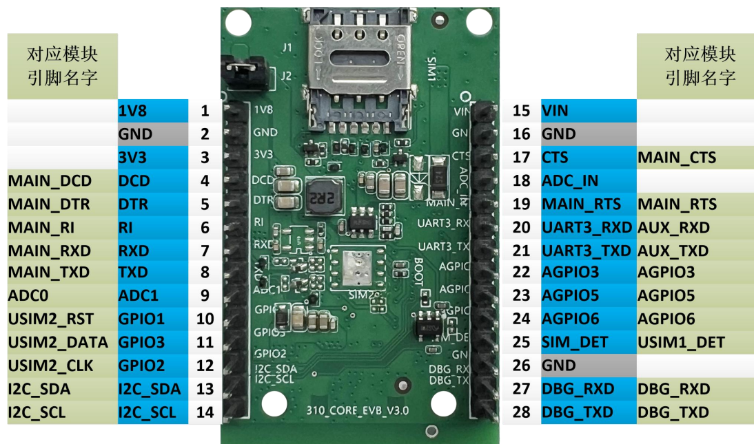
图 2-1 接口定义
