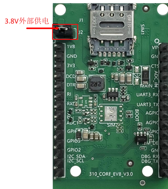
图 4-9 低功耗供电
