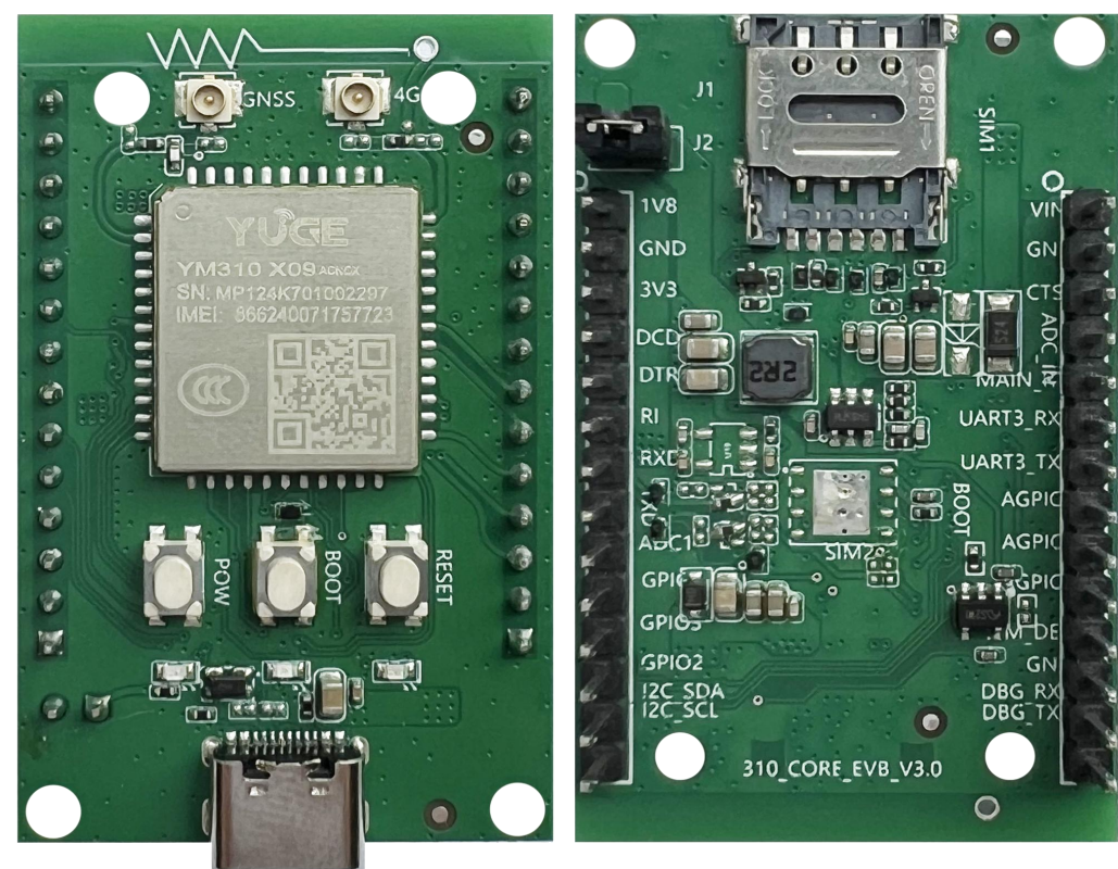
图 1-1 开发板外观图
