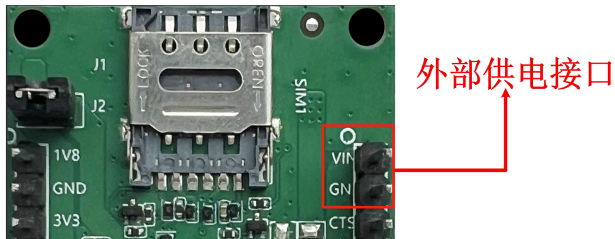
图 4-1 VIN 供电接口
