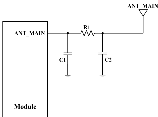
图 3-32 天线匹配电路
