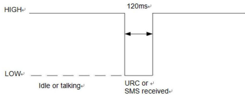
图 3-21 收到 URC 信息或者短信时 MAIN_RI 时序
