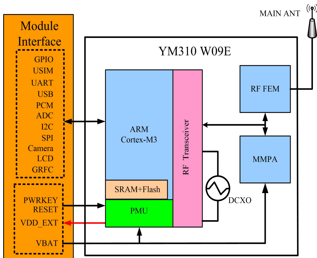
图 2-1 YM310 W09E 模块功能框图
