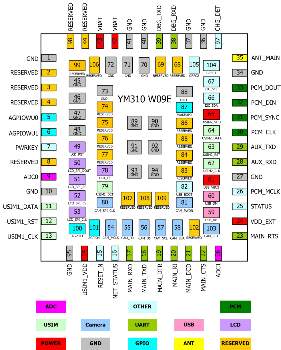
图 3-1 YM310 W09E 模块管脚分布图（TOP 透视）
