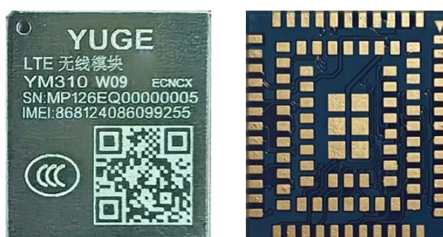
图 6-1 YM310 W09E 外观图
