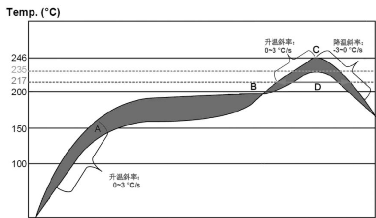
图 7-1 回流焊温度曲线图
