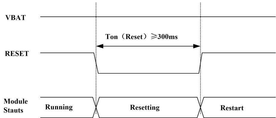
图 3-9 复位时序图
