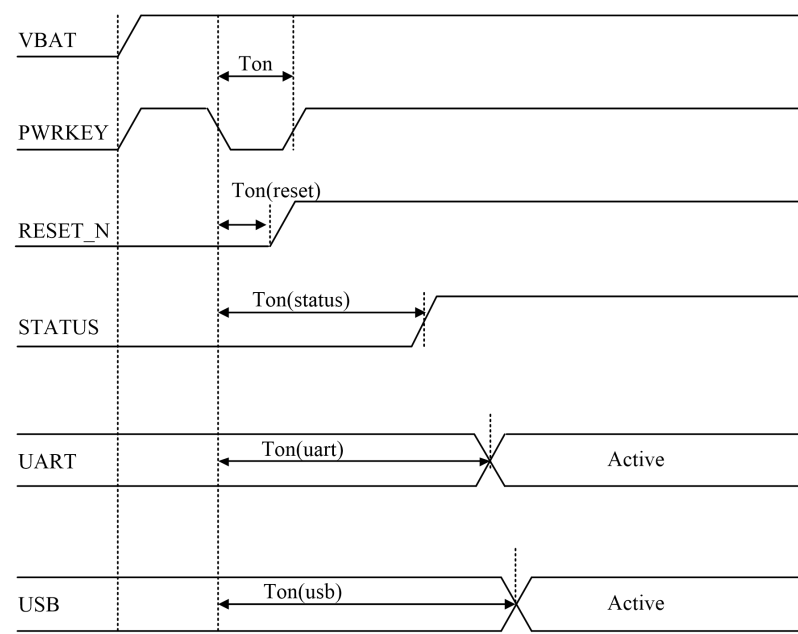
图 3-5 开机时序图
