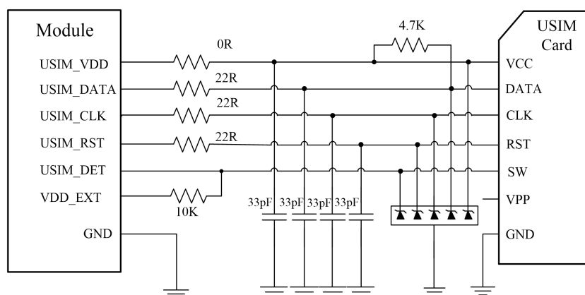
图 3-17 6pin USIM 设计参考电路图
