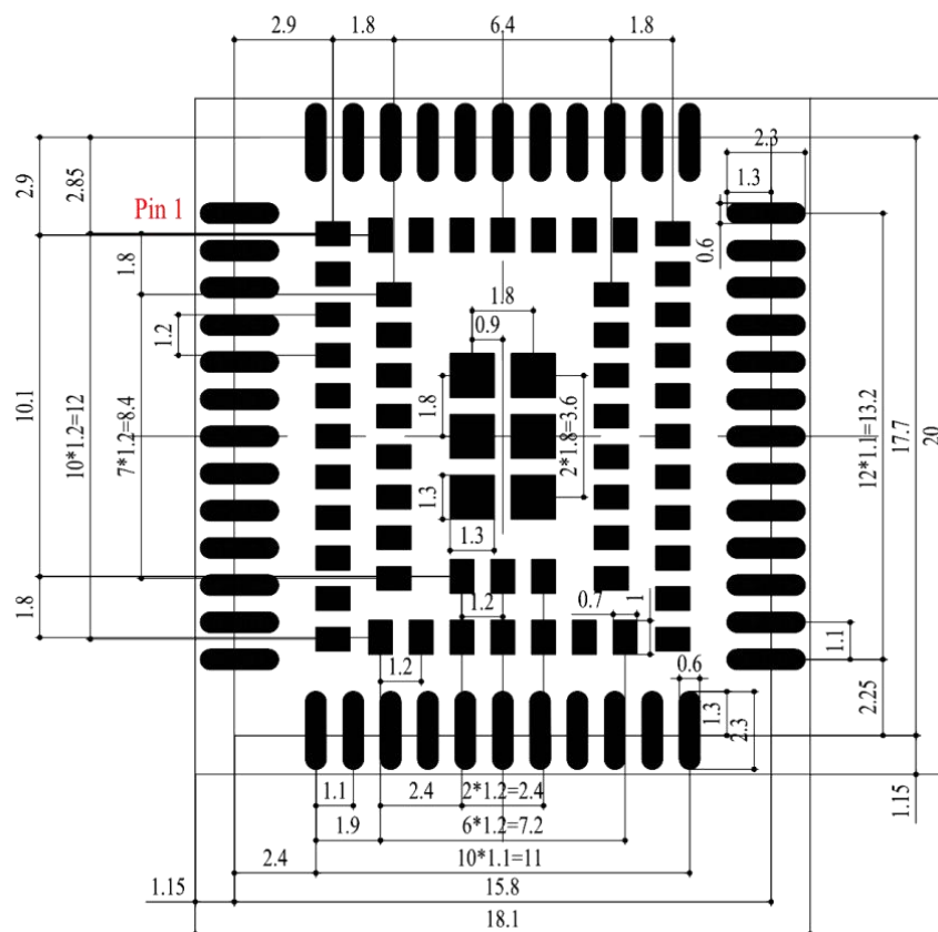
图 6-4 模块推荐封装(单位: mm)
