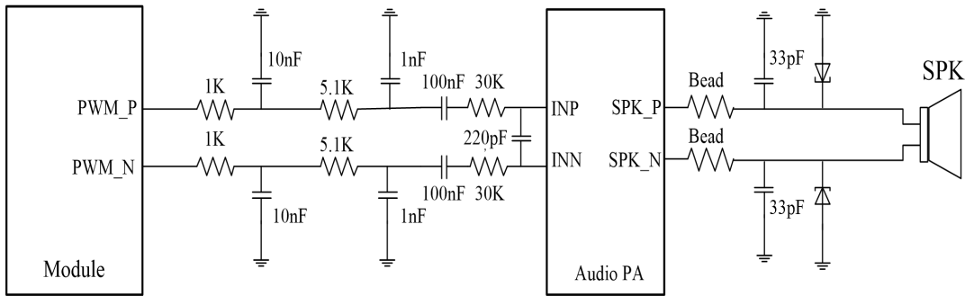
图 3-25 PWM 音频参考电路
