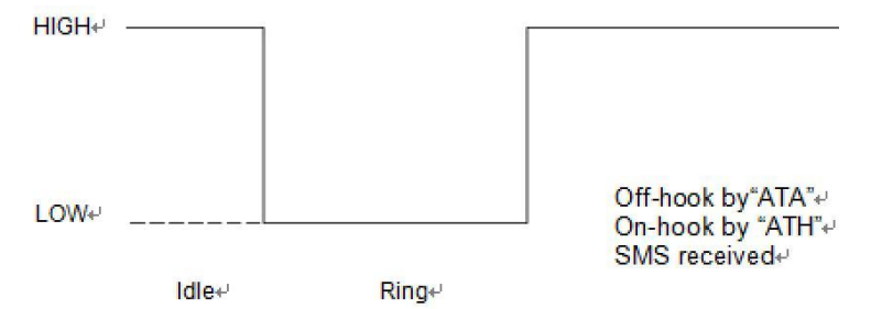
图 3-18 语音呼叫时模块用作被叫方 MAIN_RI 时序
