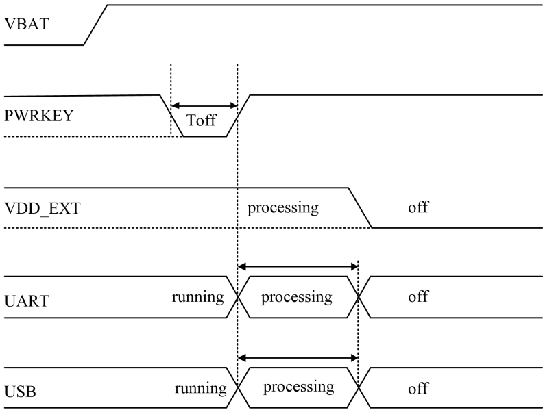
图 3-8 关机时序图
