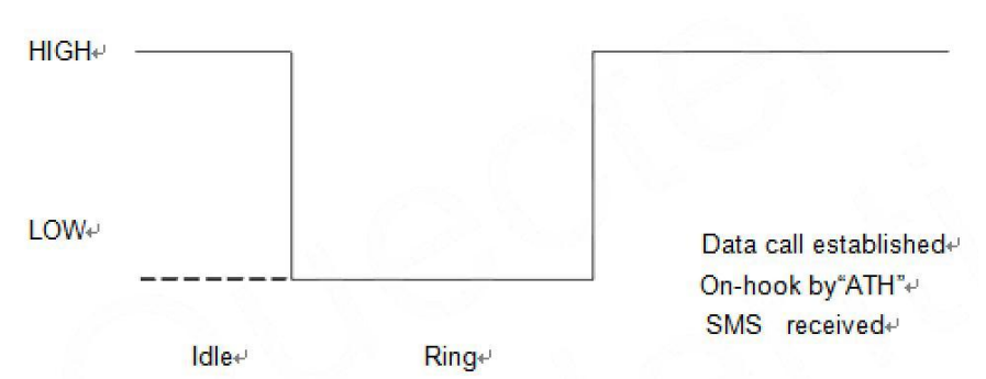
图 3-20 模块主叫时 MAIN_RI 时序
