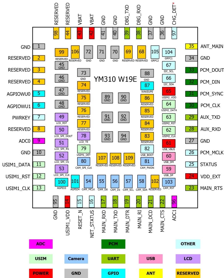
图 3-1 YM310 W19E 模块管脚分布图（TOP 透视）
