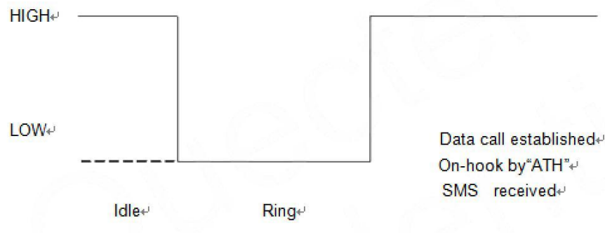
图 3-20 模块主叫时 MAIN_RI 时序
