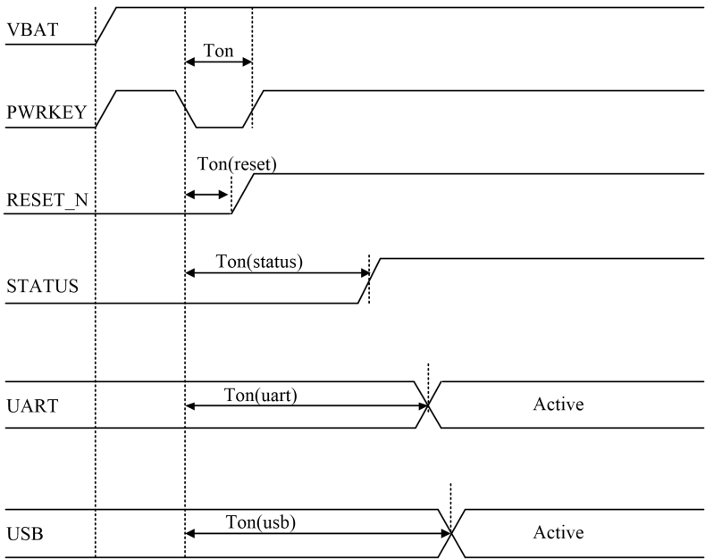
图 3-5 开机时序图
