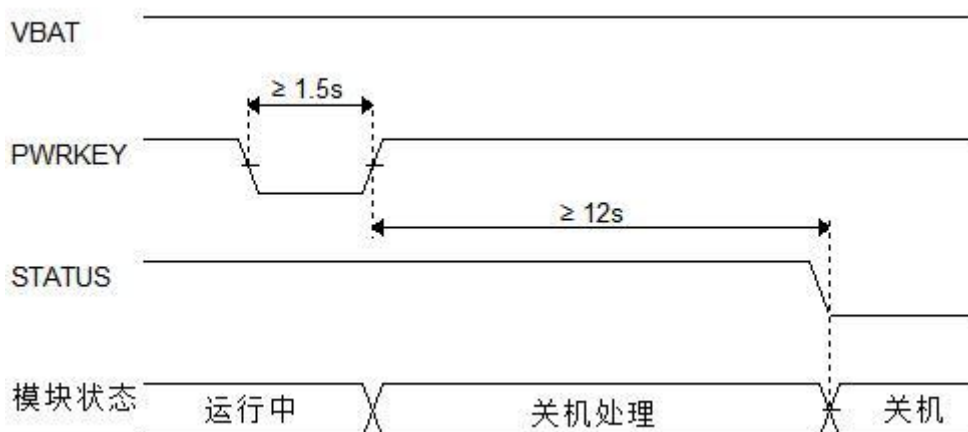
图 3-7 关机时序图
