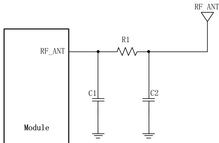
图 3-29 天线匹配电路
