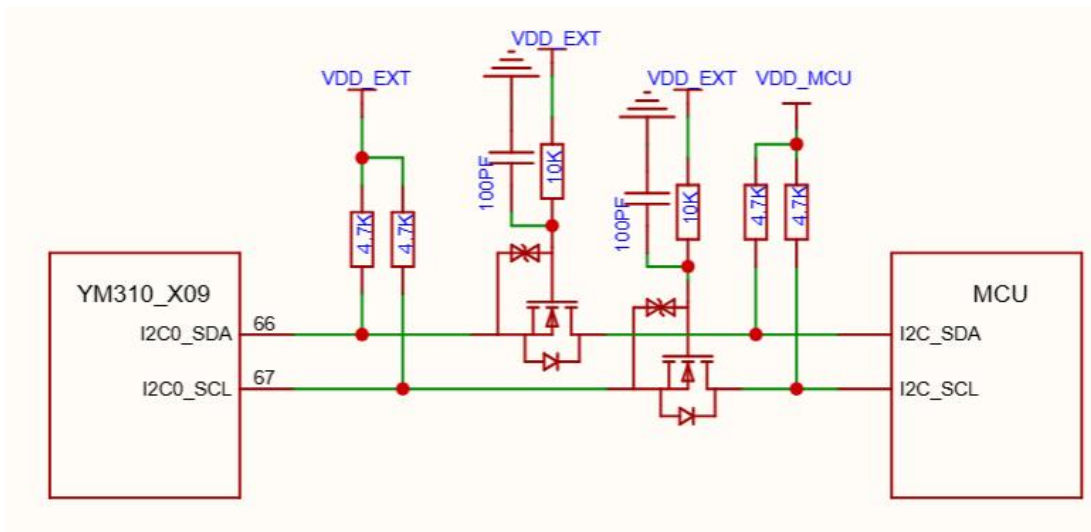
图 3-22 MCU I2C 电平转换电路
