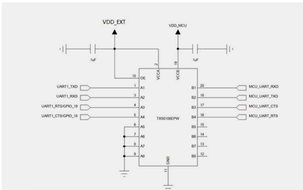
图 3-12 高波特率电平转换参考电路
