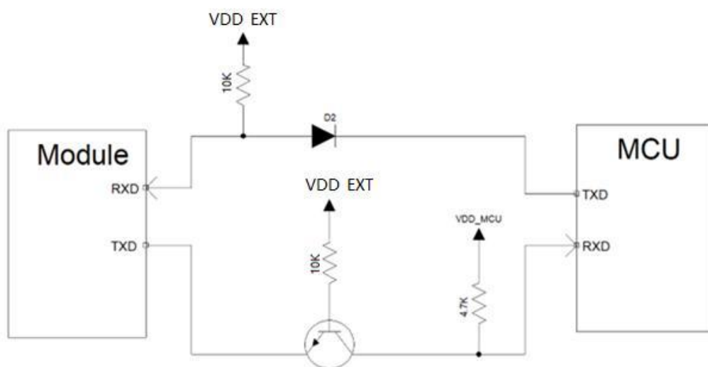
图 3-11 电平转换参考电路
