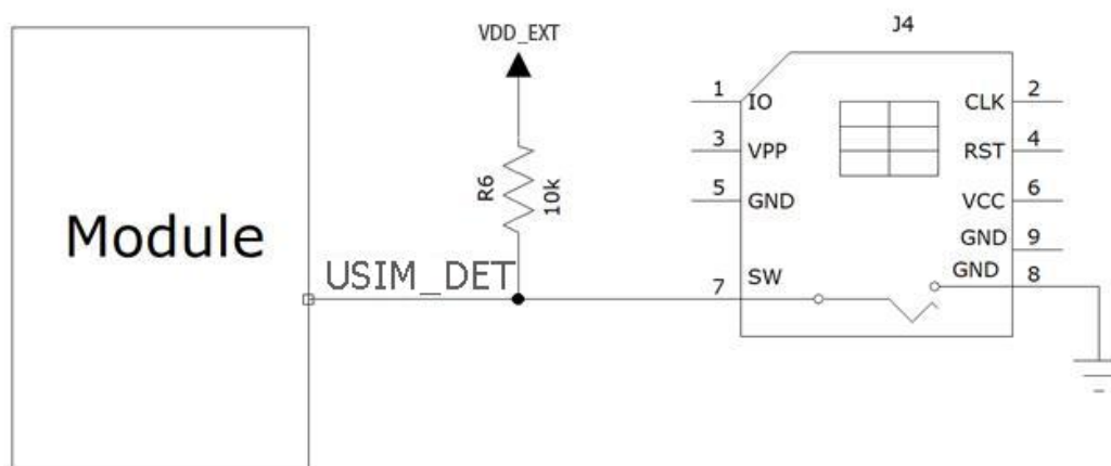
图 3-15 USIM 热插拔检测卡座参考电路图
