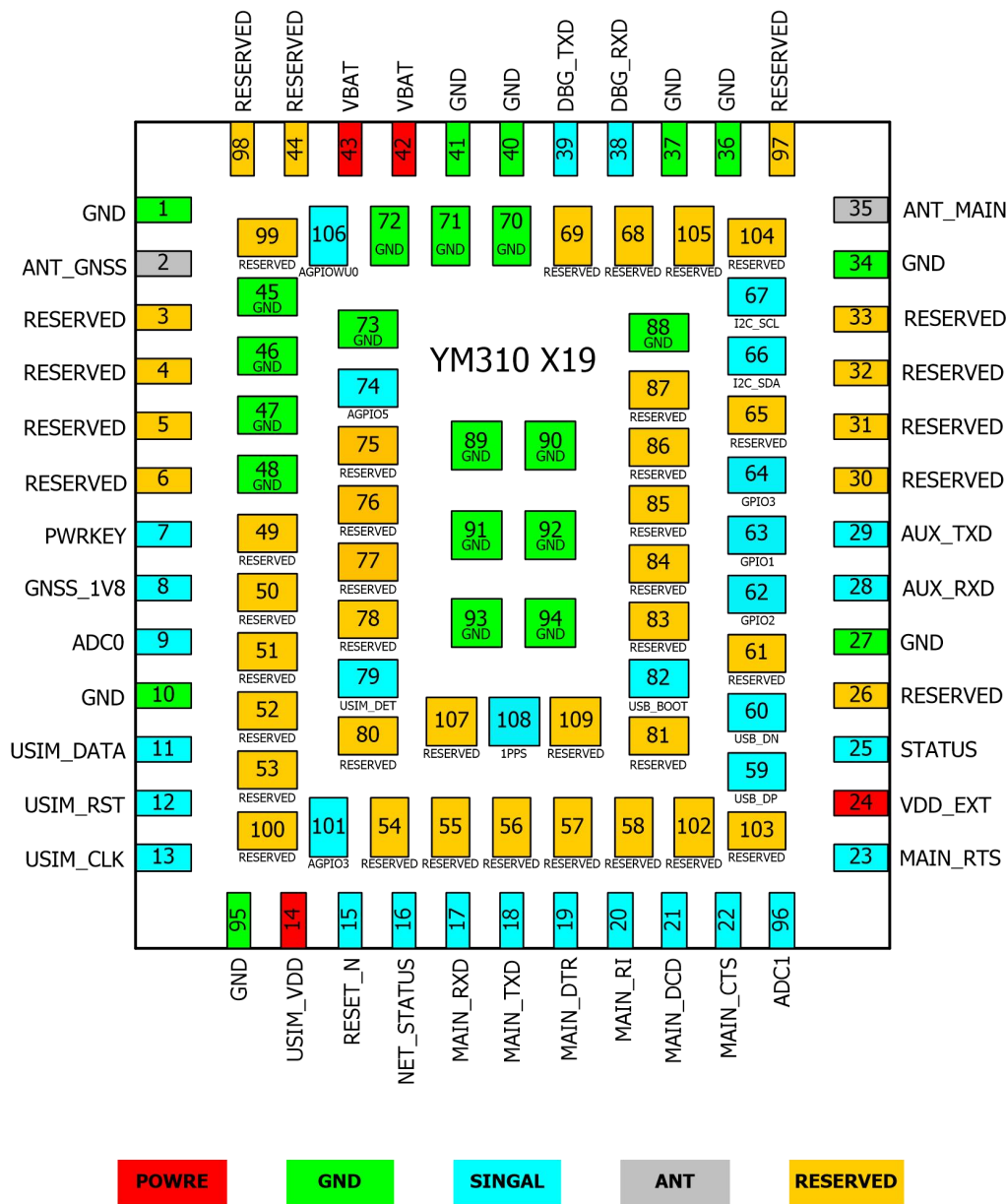
图 3-1 YM310 X19 模块管脚分布图（TOP 透视）
