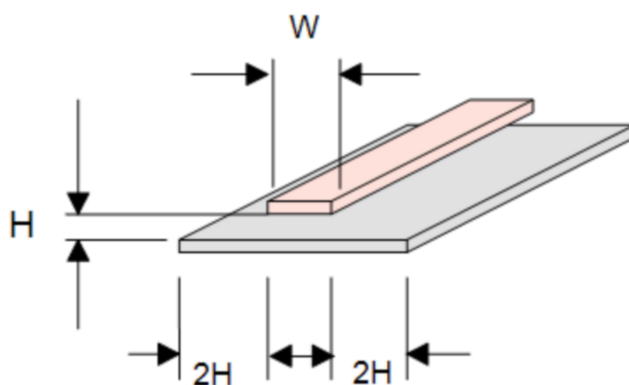
图 3-24 微带线的完整结构
