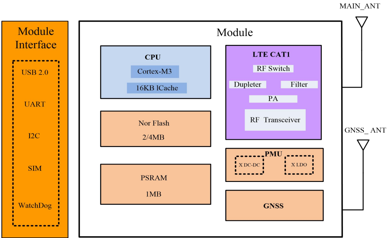
图 2-1 YM310 X19 模块功能框图
