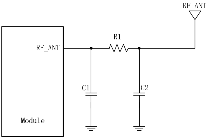
图 3-23 天线匹配电路
