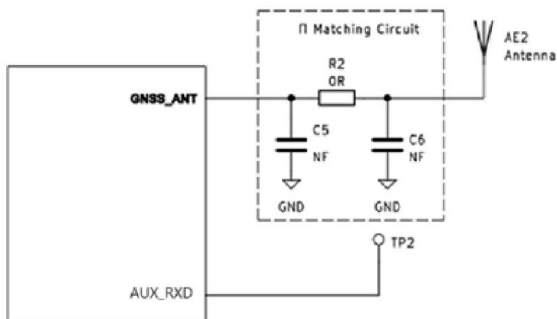
图 3-21 无源天线参考设计
