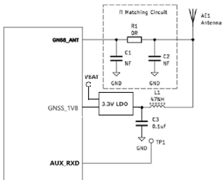
图 3-22 有源天线参考设计
