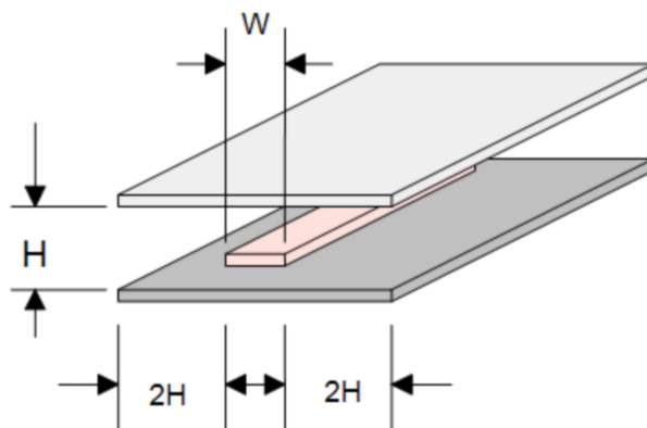
图 3-25 带状线的完整结构
