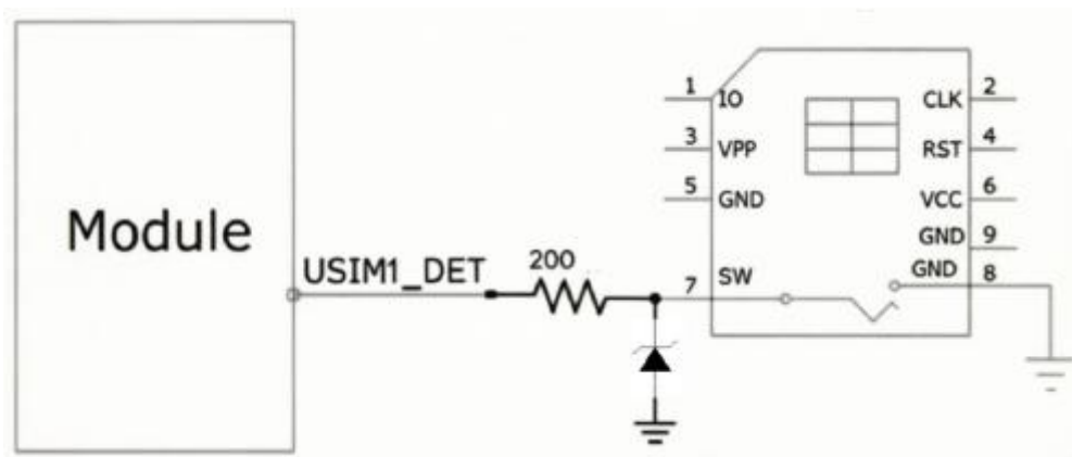
图 3-15 USIM 热插拔检测卡座参考电路图
