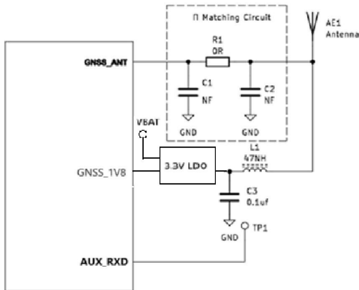
图 3-30 有源天线参考设计
