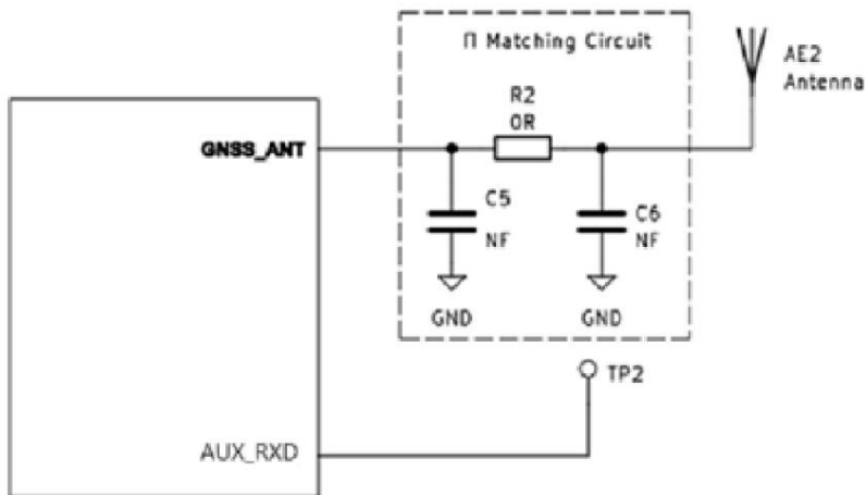
图 3-29 无源天线参考设计
