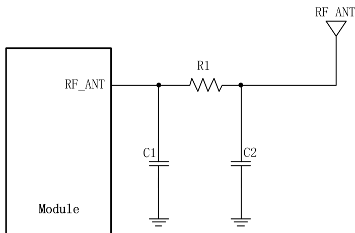
图 3-31 天线匹配电路
