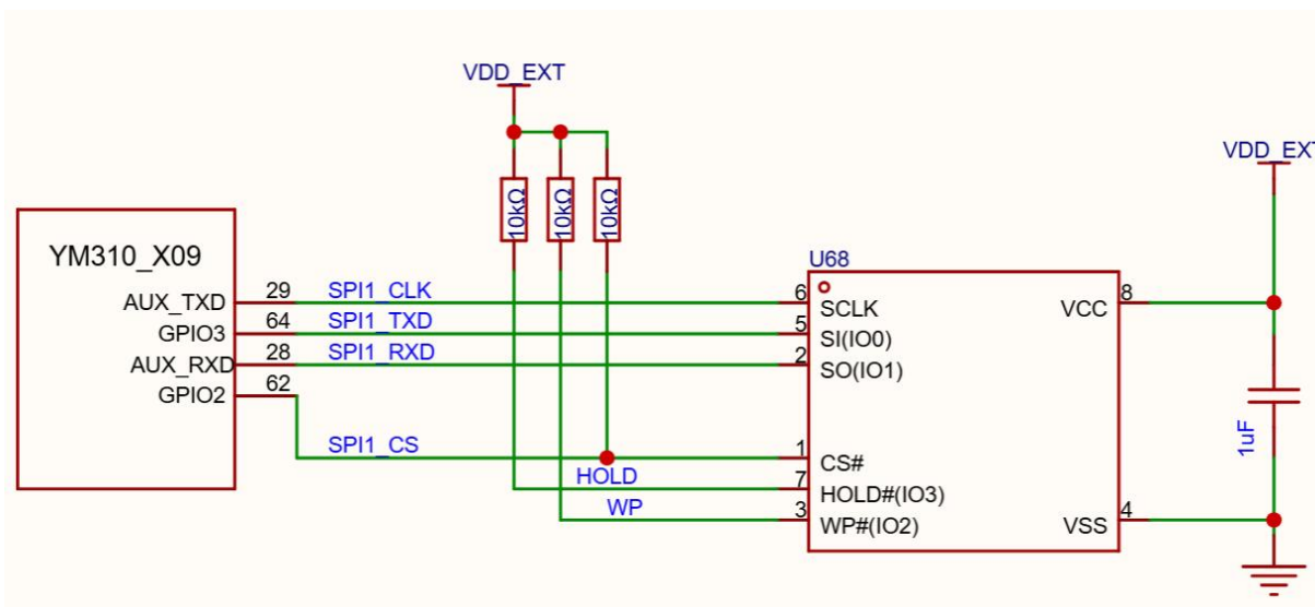
图 3-21 SPI 硬件参数参考设计
