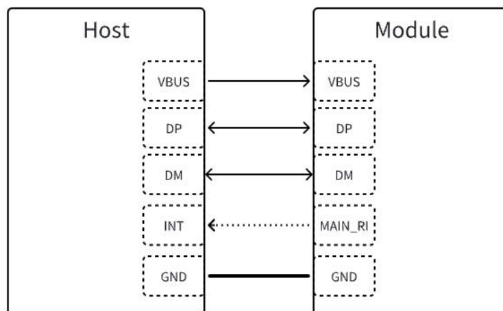
图 3-26 HOST 支持 USB 唤醒连接示意图
