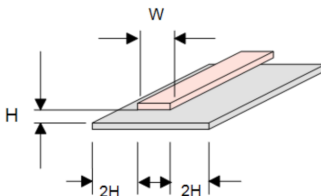
图 3-32 微带线的完整结构
