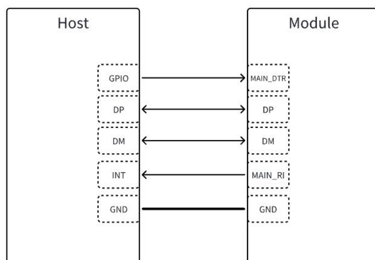
图 3-28 HOST 支持 DTR 唤醒连接示意图
