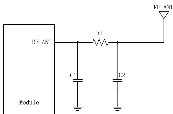
图 3-31 天线匹配电路
