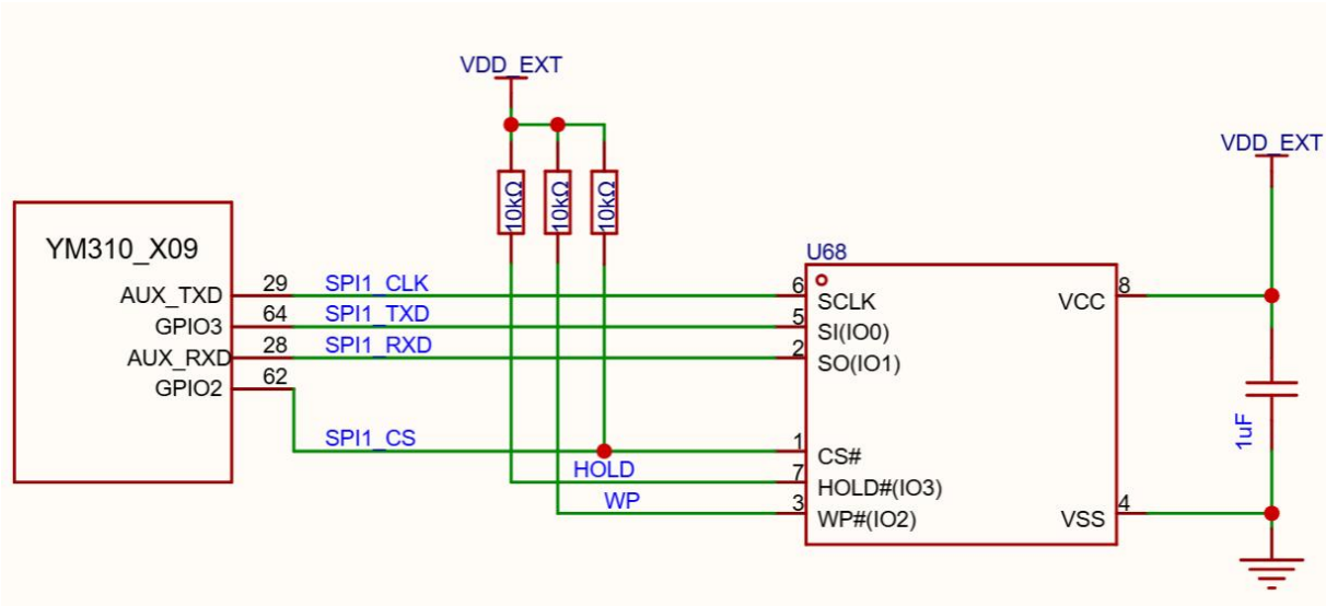
图 3-21 SPI 硬件参数参考设计
