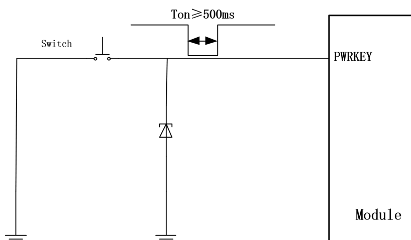
图 3-6 按键开机参考电路
