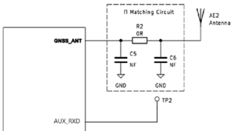
图 3-29 无源天线参考设计
