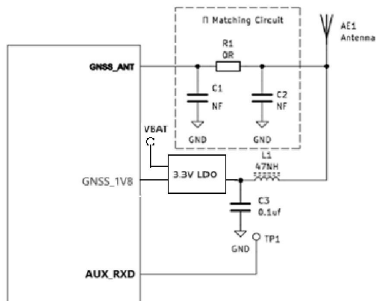
图 3-30 有源天线参考设计
