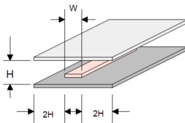
图 3-33 带状线的完整结构
